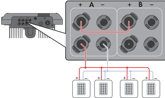
Imagen 10: Vista general de la conexión con conexión en paralelo de las entradas de CC A y B
