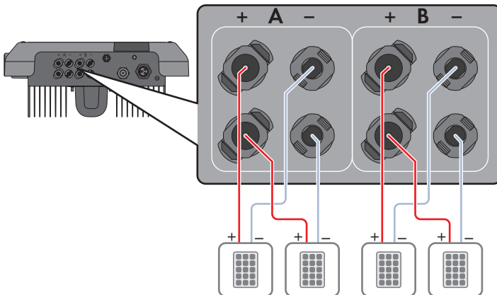
Imagen 9: Vista general de la conexión en el funcionamiento normal
