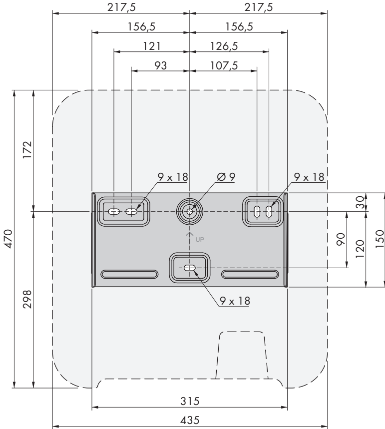
Imagen 6: Posición de los puntos de fijación (Medidas en mm)
