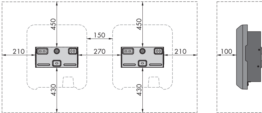
Imagen 7: Distancias recomendadas (Medidas en mm)
