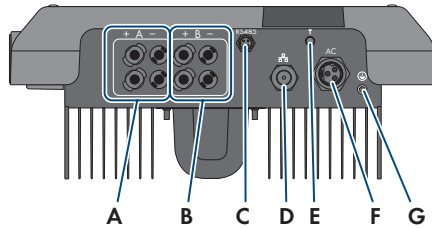
Imagen 8: Áreas de conexión de la parte inferior del inversor
