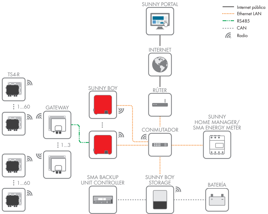
Imagen 4: Estructura de la comunicación de la planta
