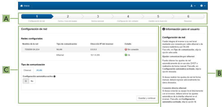
Imagen 14: Estructura del asistente de instalación (ejemplo)
