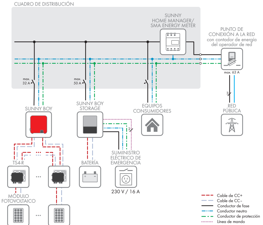
Imagen 3: Esquema de interconexión (ejemplo)
