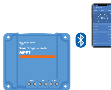
Ligação da aplicação VictronConnect através do «bluetooth» integrado
